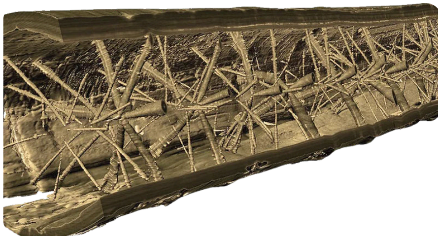
Scanner tomographique d'une grume - Illustration : Microtec
